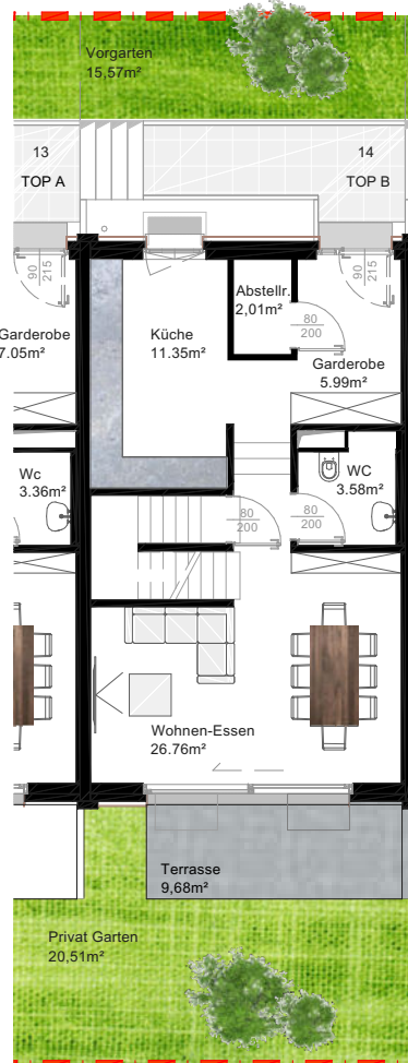
ERDGESCHOSS
