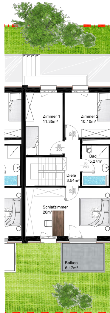
OBERGESCHOSS
